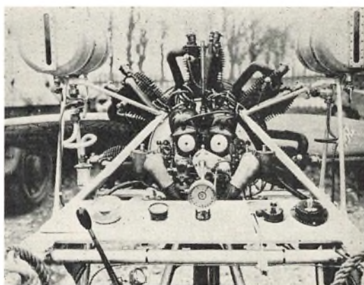
Motorgondol K—34 Motorpasserens Plads).
