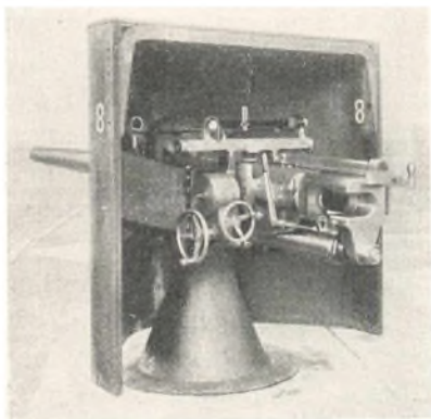
75 mm hurtigskydende Kystkanon af dansk Konstruktion og Tilvirkning.
