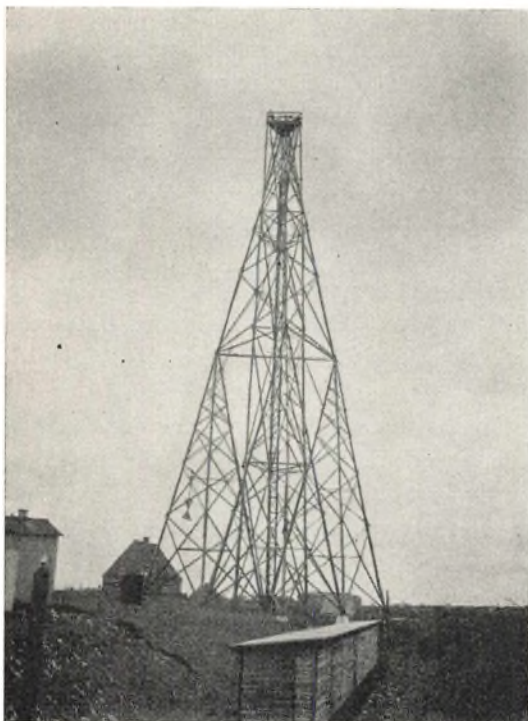
Observatoriet i Buddinge. 53 m højt Observationstaarn, rejst over trigonometrisk Station I, København.
