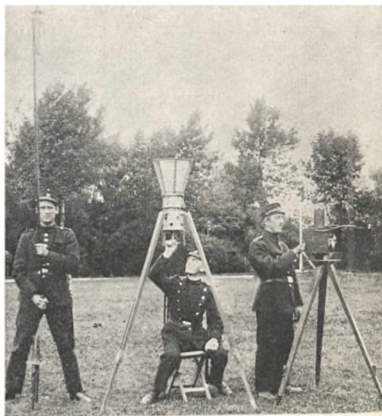
Signalering med Fakkelt (1871), Spakowskys Lanterne (1879) og Blinklanterne (1894).
