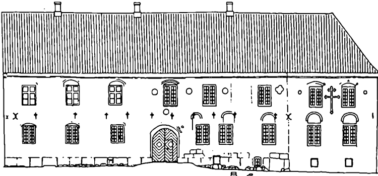
Hovedbygningens sydside, længst til højre østfløjens gavl. Opmålt af H. H. Engqvist (Nationalmuseet).
