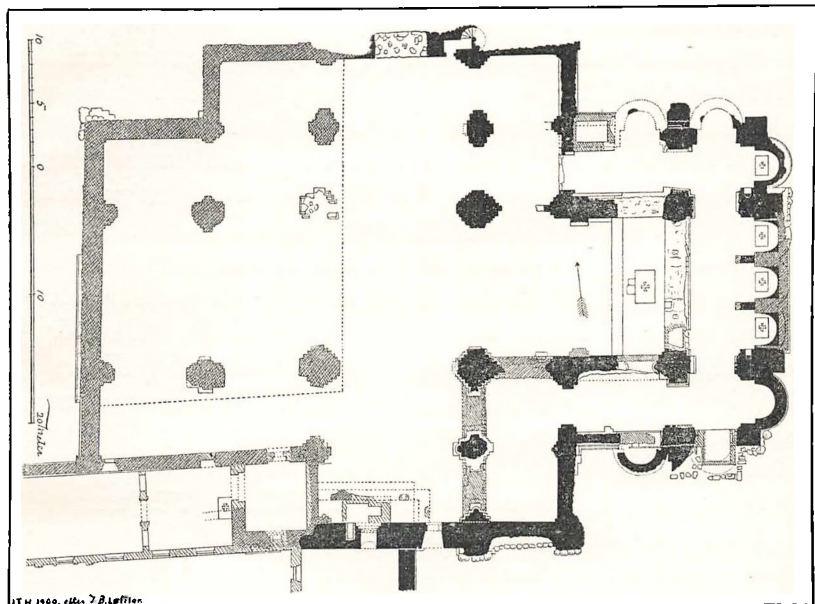
Plan af Vidskøl Klosterkirke. J. B. Løffler.
