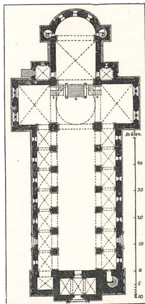
Domkirkens Grundplan. Trap
