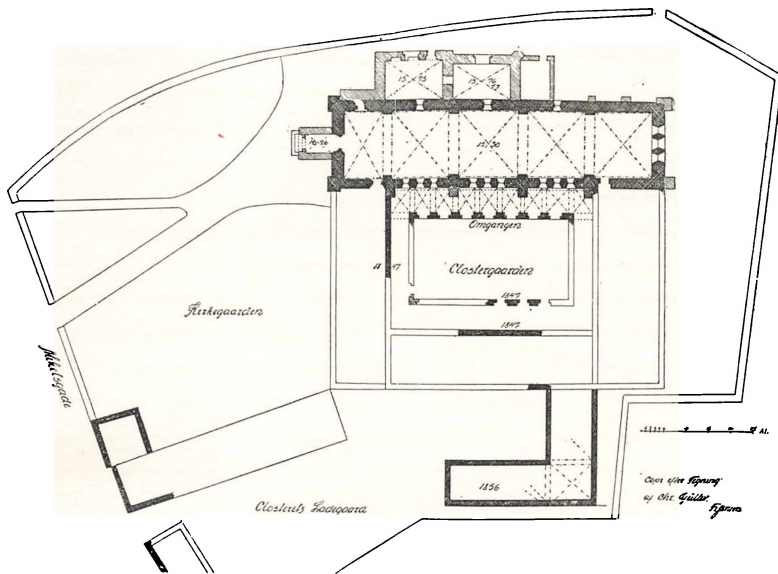
Plan af Sortebrødre Kloster. Gullev.
