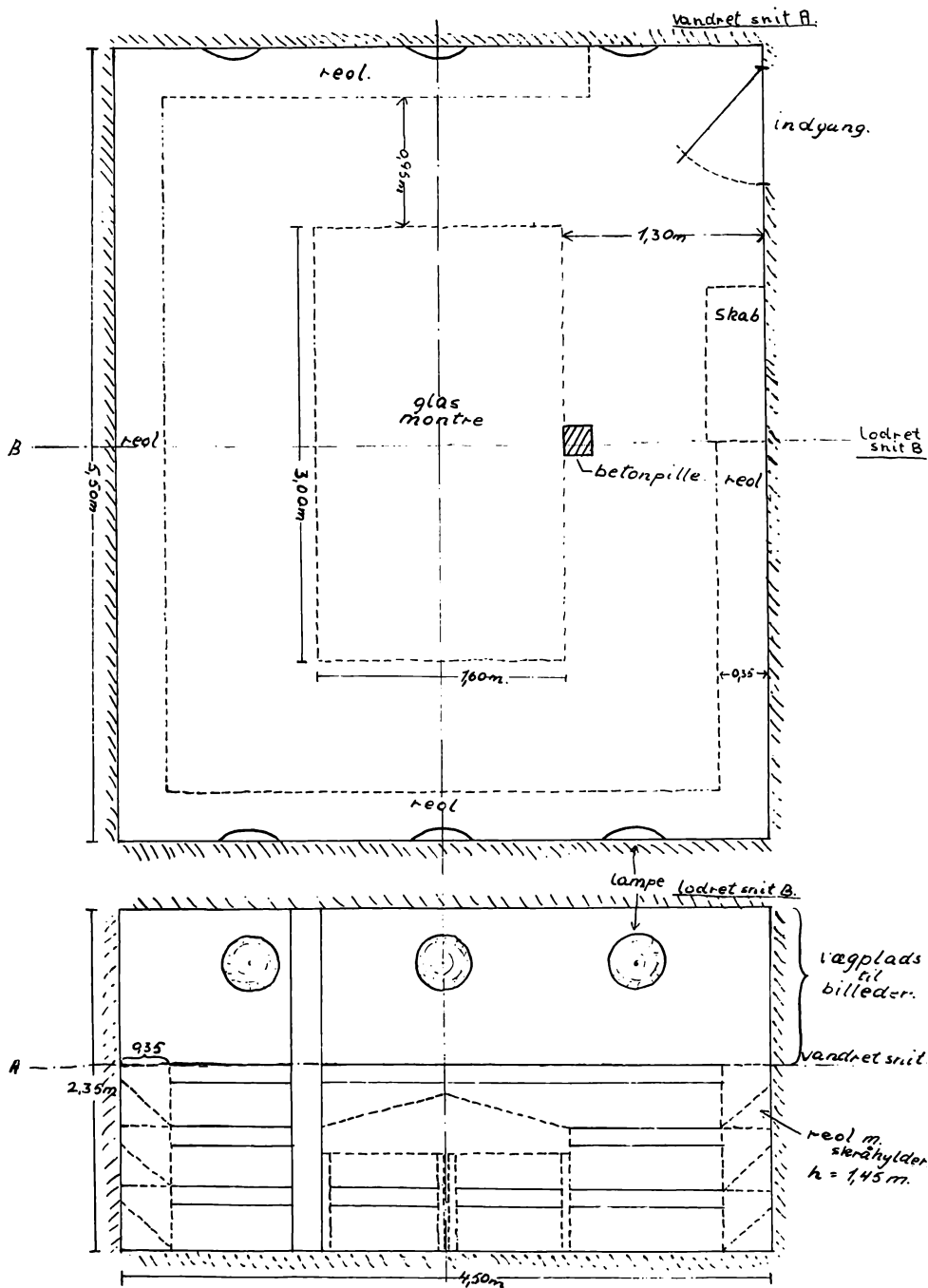
Udkast til mindestuen
