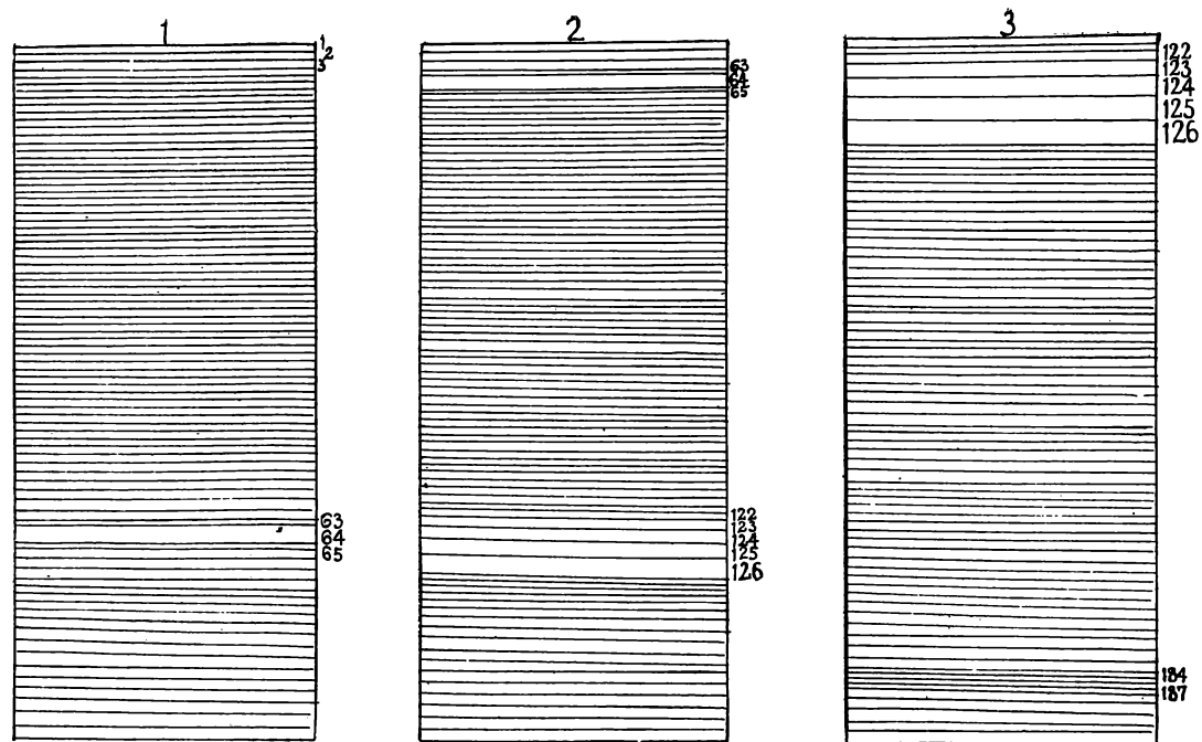
Fig. 3. Tre Profiler af lagdelt Ler. (Efter De Geer)
