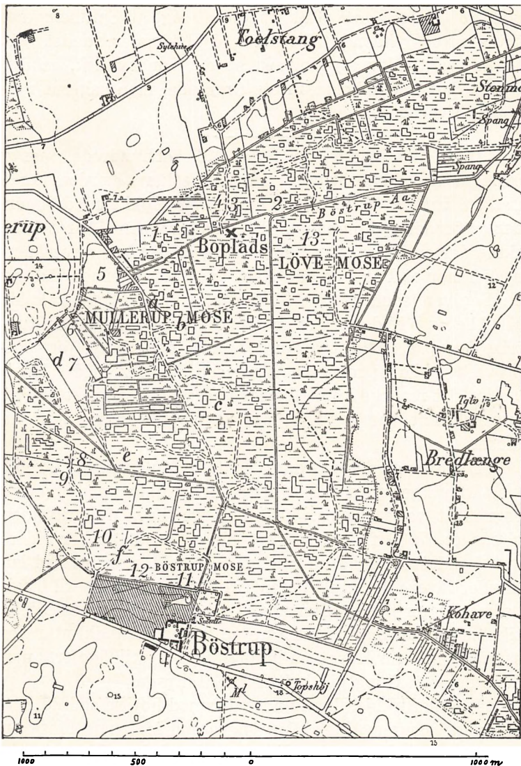
Fig. 1. Mullerup Mose. Byen til venstre. a, b og c betegner de Steder, hvor de fleste Saltbundsplanter fandtes, nu er de gaaet stærkt tilbage. Tallene viser Steder, hvor der var Stubbe. Ved 1 var de fleste (se Kortet S. 106), ved 2 Stammen, ved 3 Stubbe ved den nye Boplads, ved 4 staar enkelte endnu. Krydset viser Saraus Boplads.
