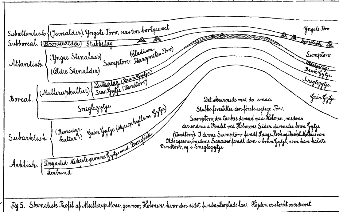
Fig. 5. Skematisk Profil af Lagene i Mullerup Mose omkring en Holm. Se Tekstens Tvivl om Tydingernes Rigtighed.
