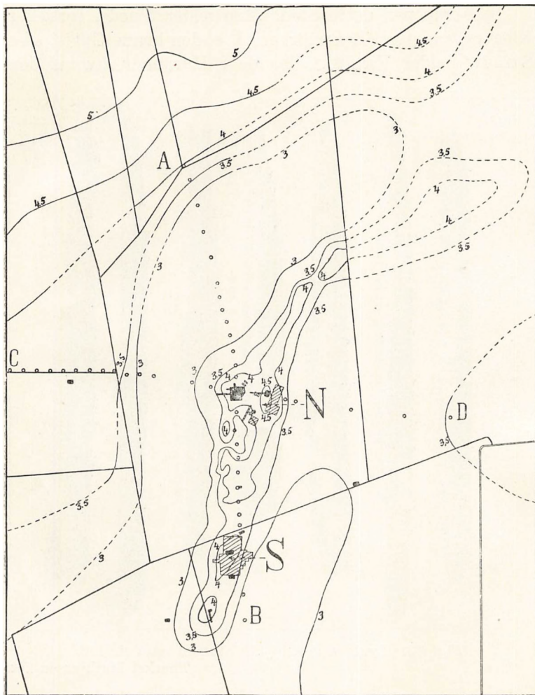
Fig. 14. Kort over Mosens Bund. Kurverne viser Sneglegytjens Overflade. De skraverede Felter viser Sarauws Udgravning (ved S) og Neergaards (v. N), de sorte Lauge Kochs og Therkel MathiasSENS.
