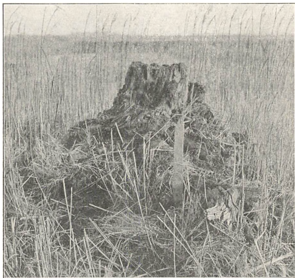
Fig. 10. Fyrrestub paa Stykke 4, Fig 1, den sværeste af alle, 40 cm høj og lige saa tyk Stamme; tilsyneladende med 2 Sæt Rødder, 4,01 m. o. H.
