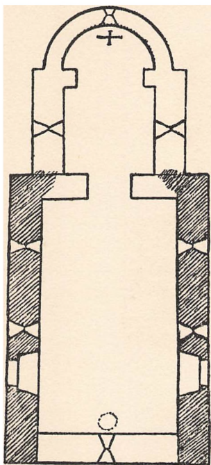
Tålbirke Kirke i sin oprindelige Grundform. De skraverede Partier findes endnu.
