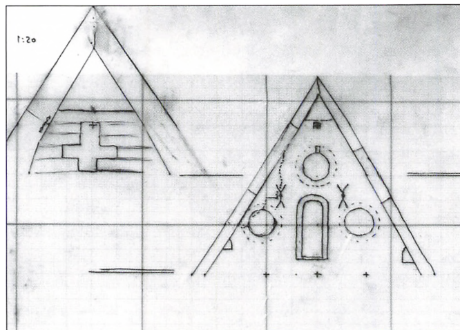
Tårnets øverste gavltrekant, udsnit af facaderegistreringens øverste del, de øverste tre stilladsk. Øverst til venstre ses detaljeregistrering af den tilbagetrukne korsformede blænding.
