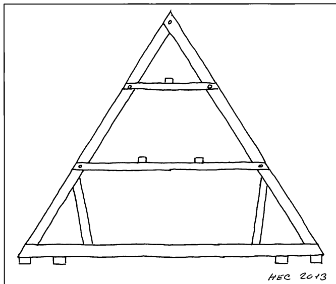
Principtegning af et af tårnets spærfag. Tegnet af Hans Erik Christensen 2013.
