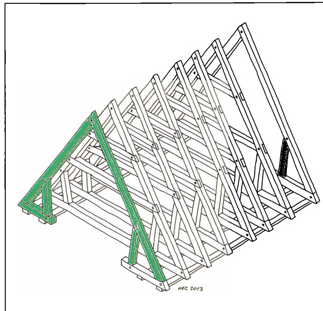
Principtegning af hele tårntagværkets konstruktion. Tegnet af Hans Erik Christensen 2013. Efterfølgende er de dele, der er udtaget til datering markeret med farve og x.nr.
