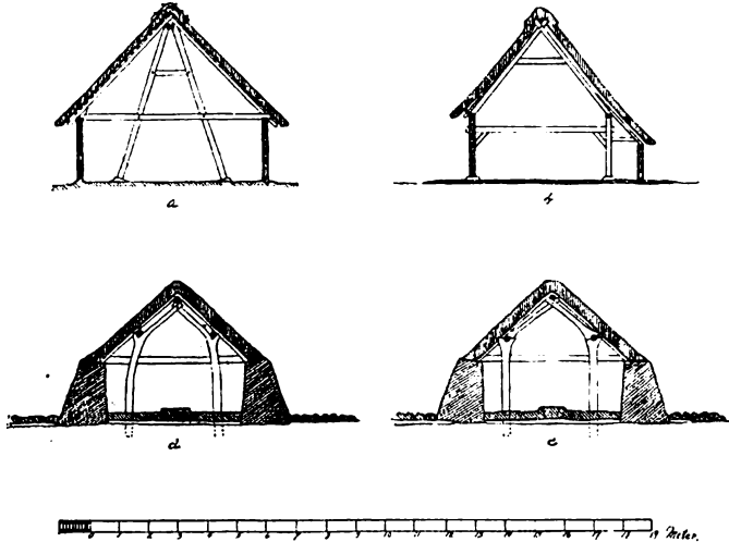
Fig. 3. — Tværsnit af Sule- og Udskudshuse, samt Forsøg paa en Rekonstruktion af Tværsnittet af et Hus fra den yngre Oldtid (Fig. 2, Huset A). a. Sulehus fra Salling. b. Højremshus fra Himmerland. c. og d. Rekonstruktioner af Tværsnittet af Oldtidshuset.
