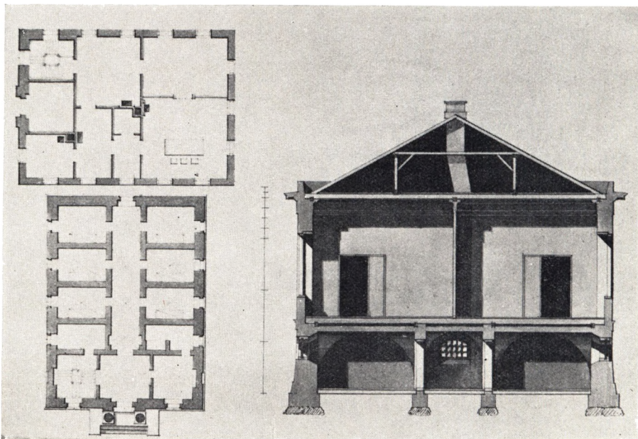
Grundplan og Gennemsnit af Ting- og Arresthus i Sorø (?)
