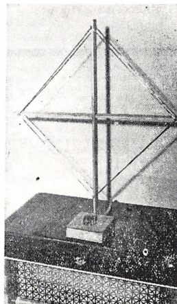
Rammeantenne.
