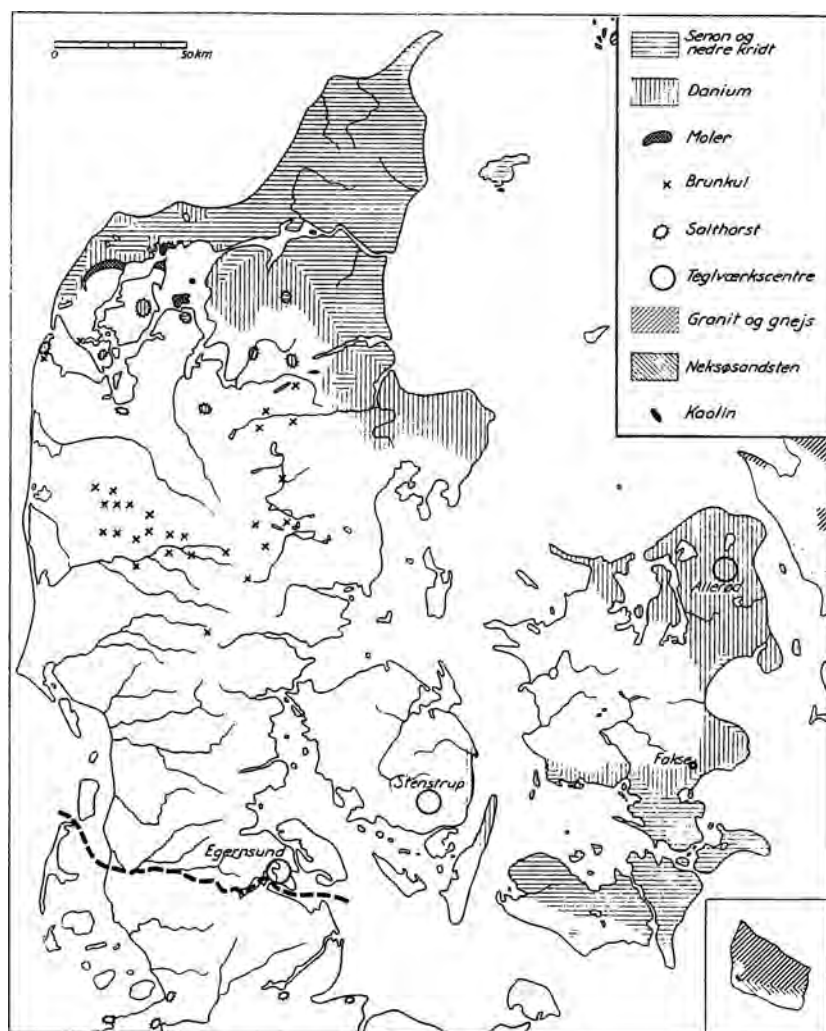
De vigtigste udnyttede mineraler i Danmark.
