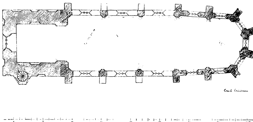
Fig. 37. Grundplan af St. Peders Kirke.
