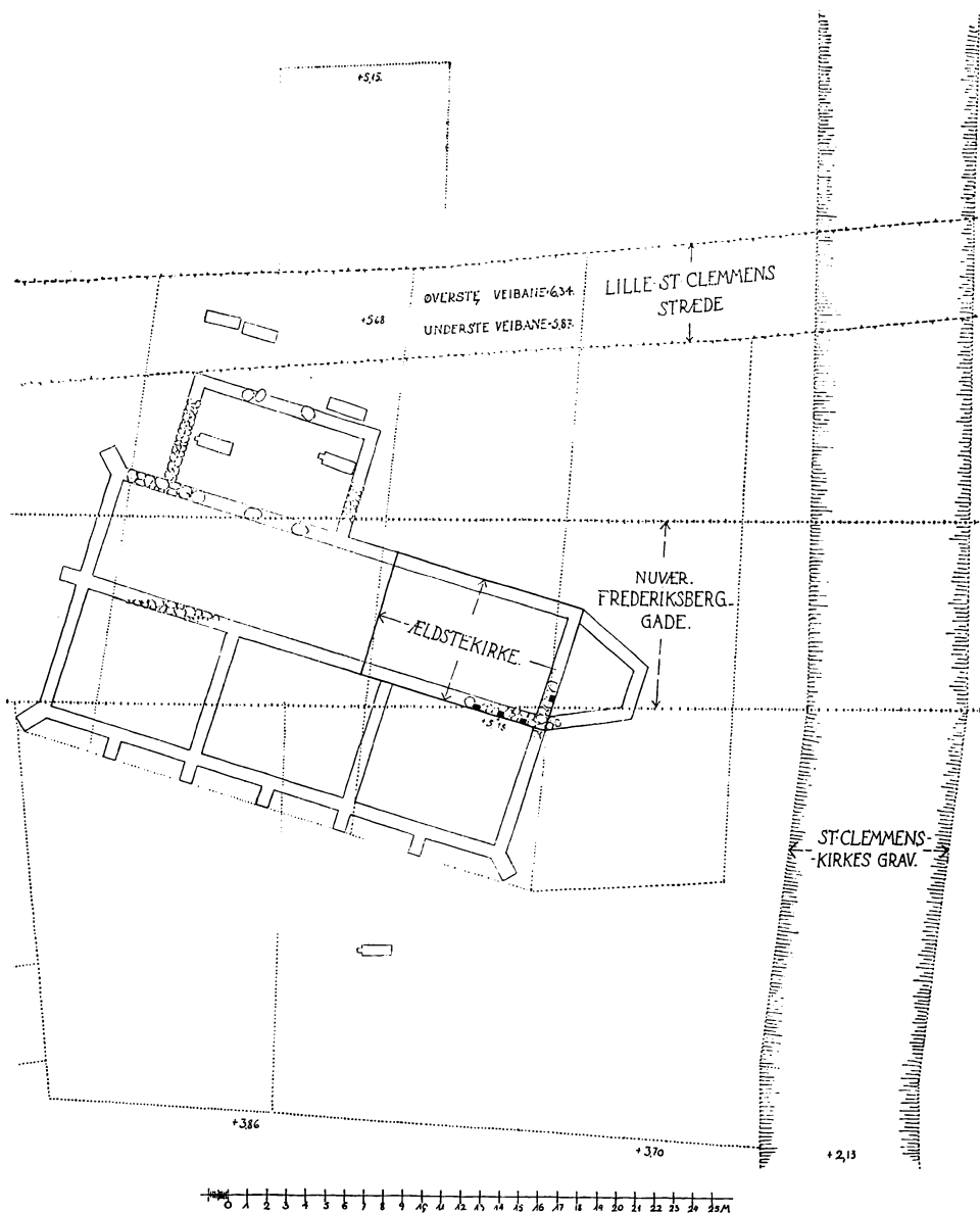
Fig. 24. Grundplan af St. Clemens Kirke.
