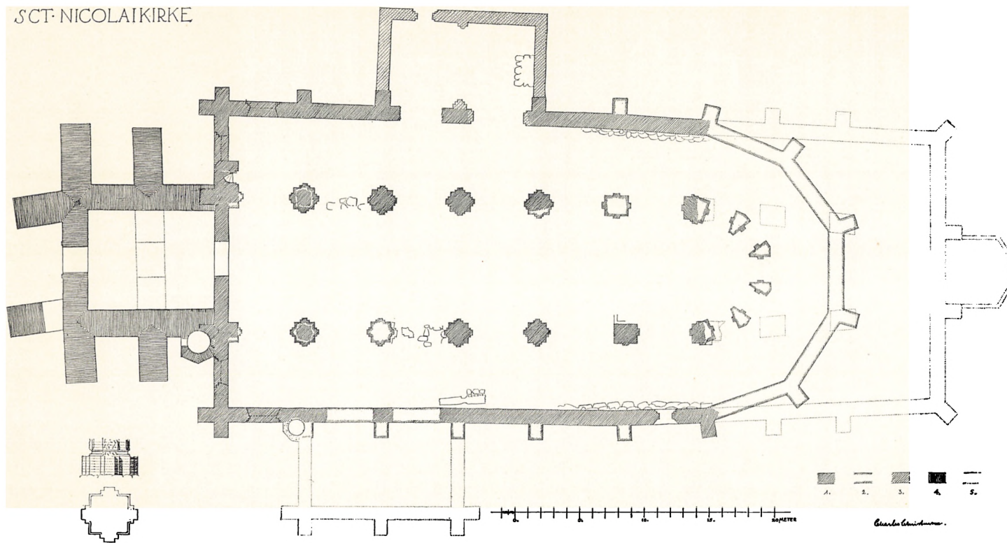
Fig. 35. Grundplan af St. Nicolaj Kirke.
