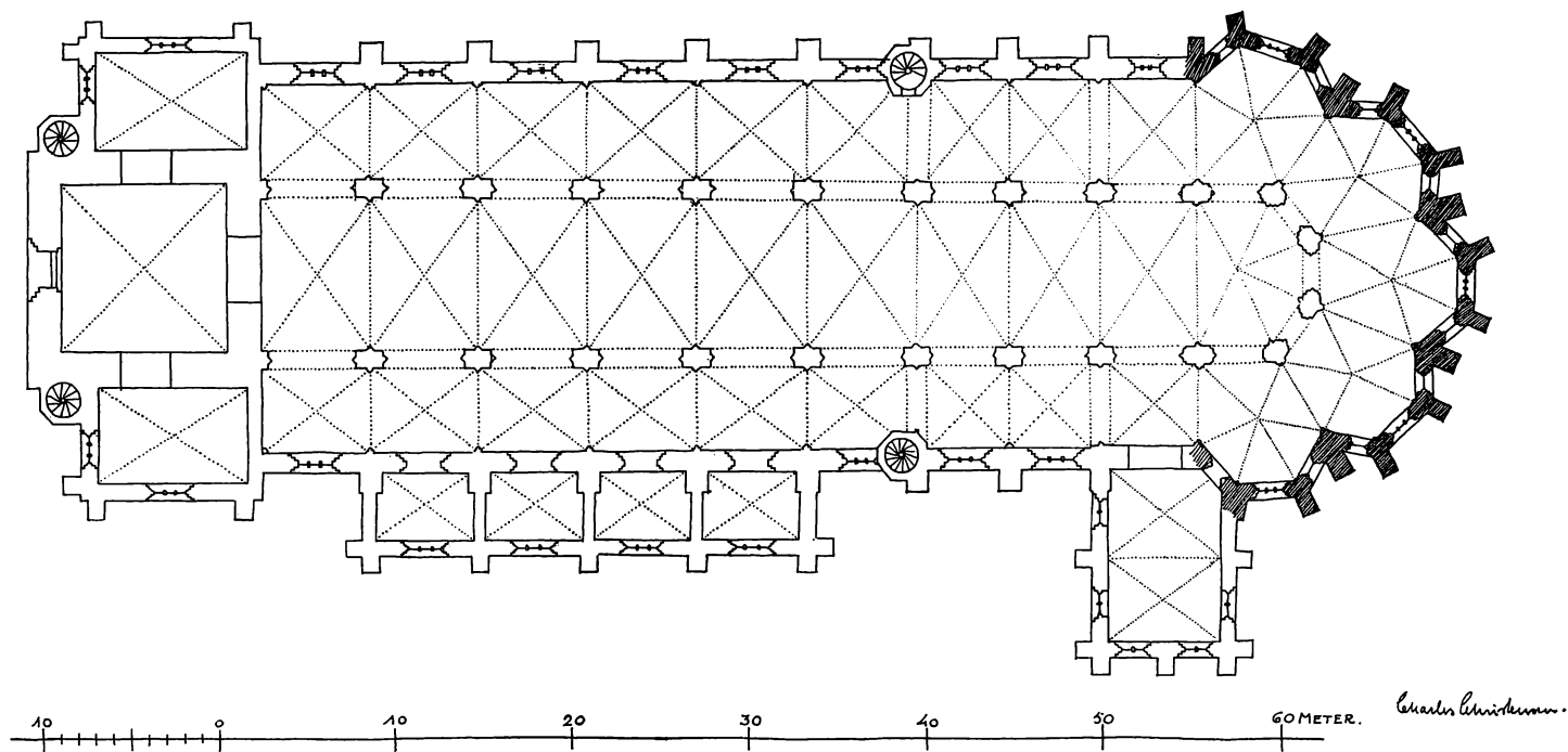
Fig. 29. Rekonstruktion af Vor Frue Kirkes Grundplan ved Slutningen af Middelalderen.
