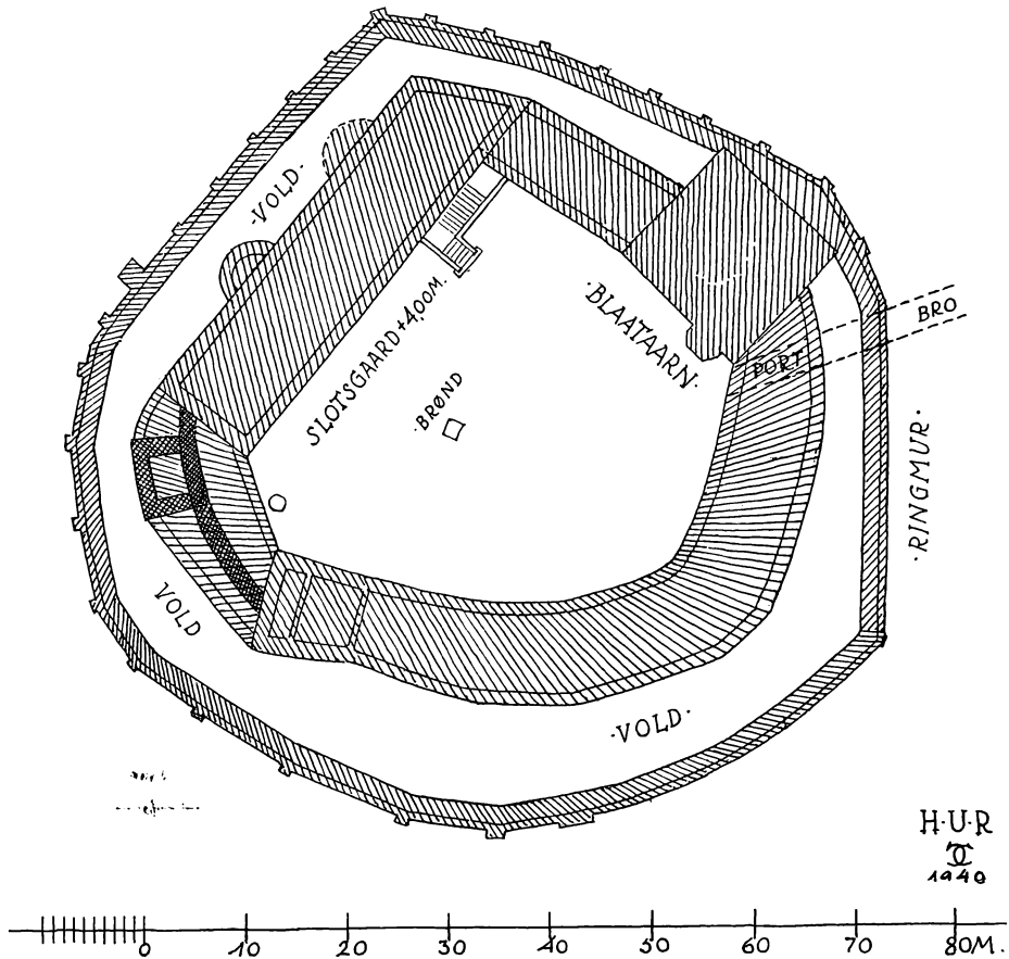
Fig. 14. Grundplan af Slottet efter 1369.
