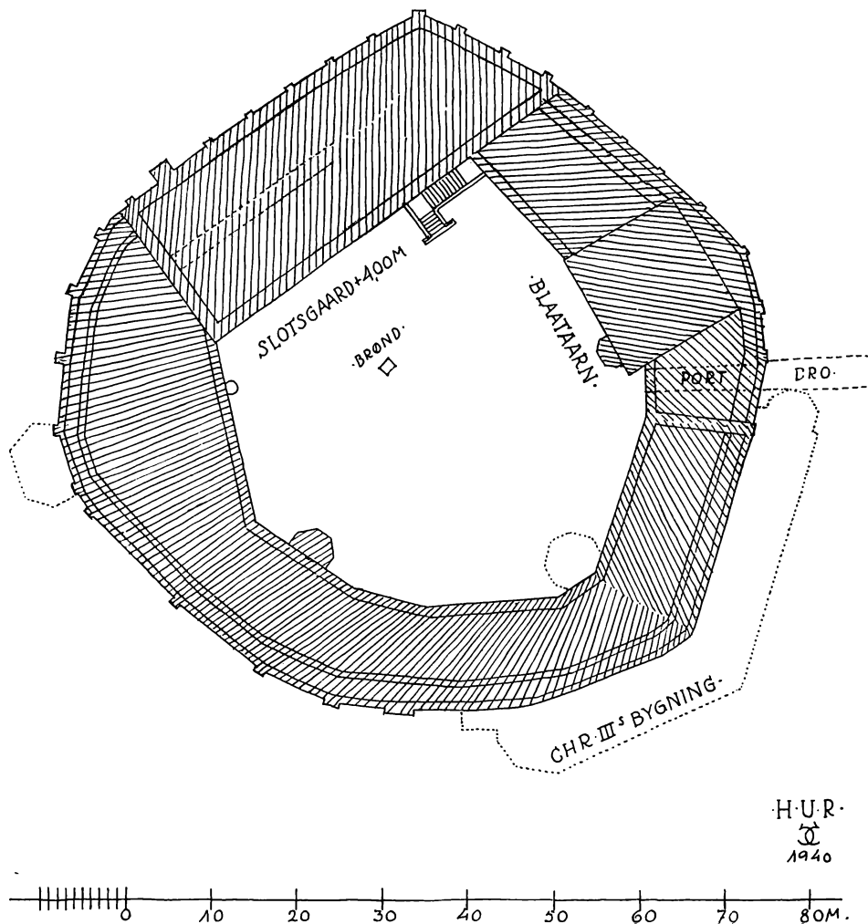
Fig. 19. Grundplan af Slottet i Slutningen af Middelalderen.
