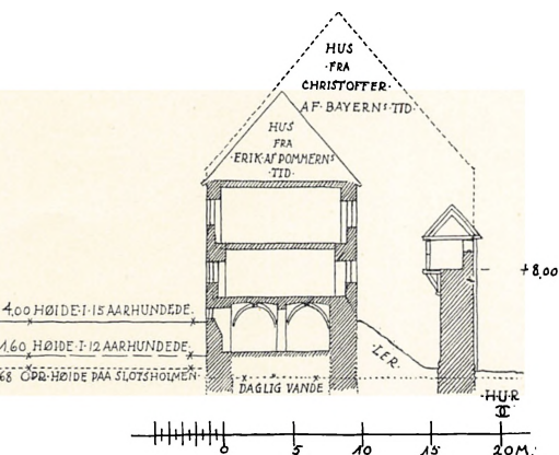
Fig. 12. Rekonstruktion af Tindemuren udfor Riddersalen.
