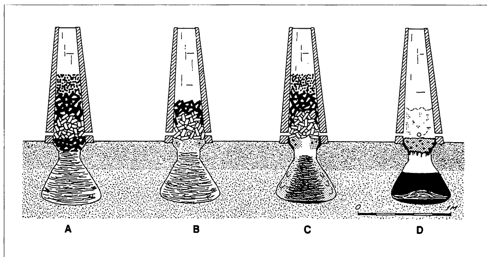
Fig 3. Tværsnit af jernudvindingsovne, fire stadier i jernudvindingen.
