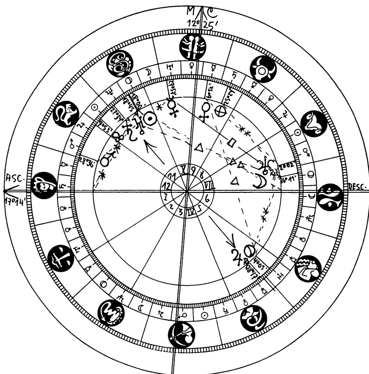
Radixhoroskop for Frederik II, født 1. juli 1534 kl. 9.30 lokal tid = 9.00.26 GMT (Jul. Dato 2.281.532,9) i Haderslev 55° 15' N, 9° 29' Ø. Regiomontanus system.
