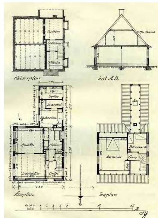
Plantegning af de første landarbejderboliger i Danmark
