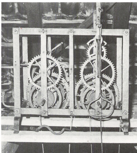
Tårnurværket fra Ørsted kirke med stenlodder og pendul, som i 1961 blev overgivet til kulturhistorisk museum i Randers Foto: Kirsten Nijkamp.
