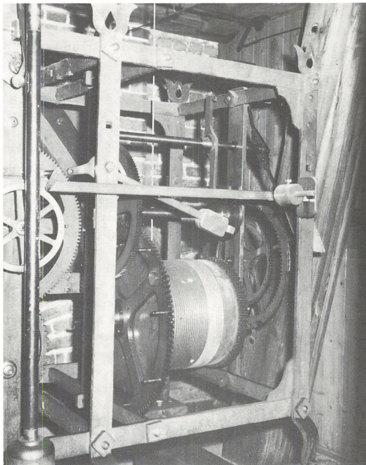
Sct. Mortens kirkes tårnurværk, Randers. Fot. Hans Stiesdal. (Randers Lokalhistoriske Arkiv).
