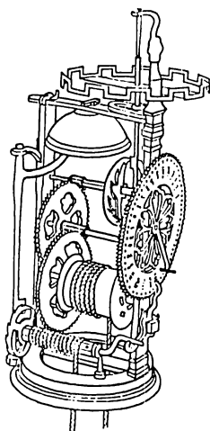
Vækkerur, som blev brugt af munke ca. 1460
