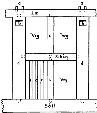
Fig. 3. Skematisk Tegning af Bindingsværk. aa. Plads til Sparrer. bb. Huller til Bjælke. cc. Doppe. dd. Stålp. ee. Hæl.
