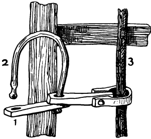
Fig. 27. Kokloe. Original i Dansk Landbrugsmuseum. 1. Nål. 2. Bøjl. 3. Rænepæl. (Naar Bøjlen er lukket, ses Enden nedenunder Naalen.)
