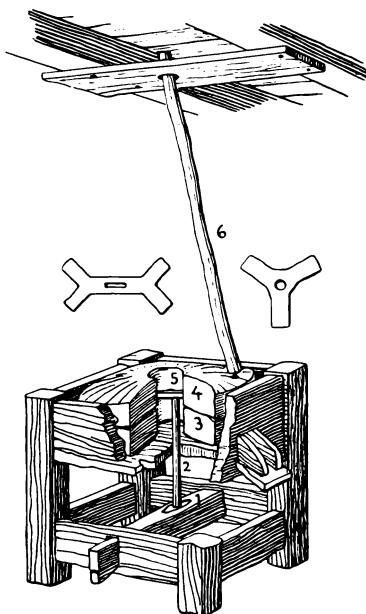
Fig. 11. Håndkværn. (Stykke af Bordet og Stener for Anskueligheds Skyld udtaget.)
