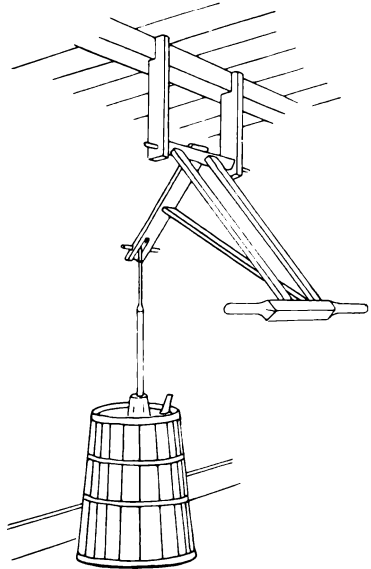
Fig. 37. Venkerne. Original i Dansk Landbrugsmuseum.
