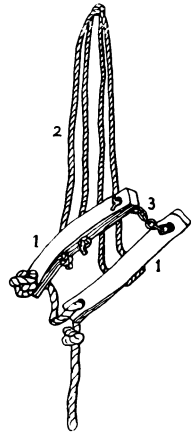
Fig. 29. Klappgremme. Original i Dansk Landbrugsmuseum. 1. Klaptræ. 2. Hostolerev. 3. Jærnlænke.
