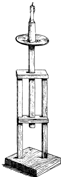
Fig. 13. Lysefod af Træ. Original i Dansk Landbrugsmuseum.
