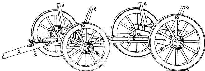
Fig. 31. Lundstikkevogn. Original i Dansk Landbrugsmuseum.
