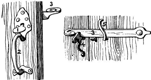
Fig. 5. Klenke. 1: Klenkejækk. 2: Håntøj. 3: Klenke. 4: Klenkehakk. 5: Klenkefall.
