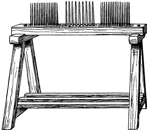
Fig. 65. Hørrive. Original i Dansk Landbrugsmuseum.
