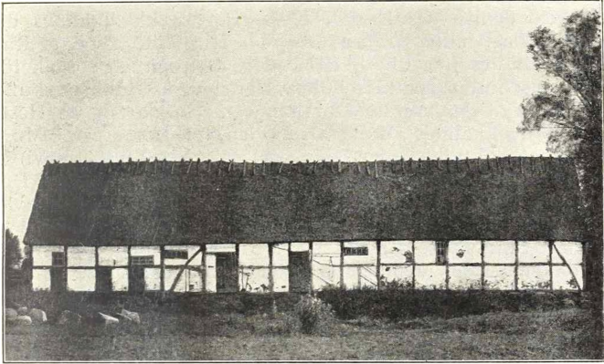
Fig. 19. Klokkergaardens nørre Længe set fra Nord. De fire østlige Fag er yngre.
