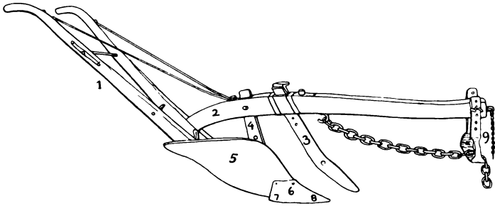
Fig. 54. Plo. Original i Dansk Landbrugsmuseum.
