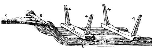
Fig. 33. Slæc. Tegnet efter Lars Rasmussens Anvisning. 1. Slæmee. 2. Å \eta neng. 3. Slææne. 4. Kæpp. 5. Hals. 6. Stang.
