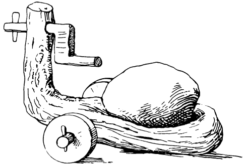
Fig. 75. Revvon. Tegnet efter Lars Rasmussens Anvisning.
