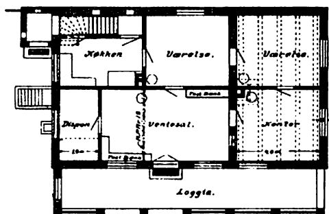
Stueplan.
