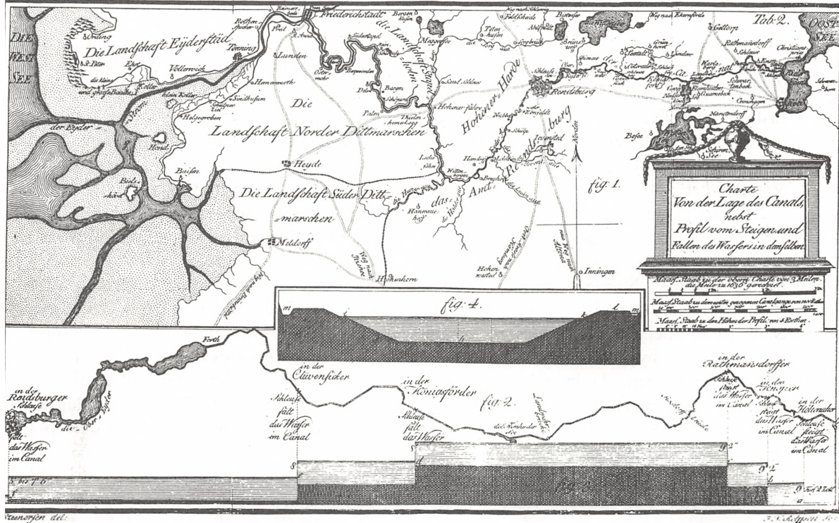
Gammelt kort over Ejderkanalen fra Holtenå til Rendsborg, hvor kanalen forbindes med Ejderfloden. På fig. 2 er sluserne i kanalen indtegnet, på fig. 3 ses de tilsvarende vandstandshøjder, og endelig fremgår kanalprofilen af fig. 4. (Efter Georg Bruyn. 1784).
