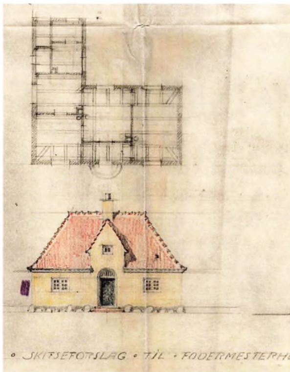
Skitse tegning til Barfredshøjs fodermesterhus udarbejdet i 1917 af arkitekt Gerhardt Poulsen (1883-1918).
