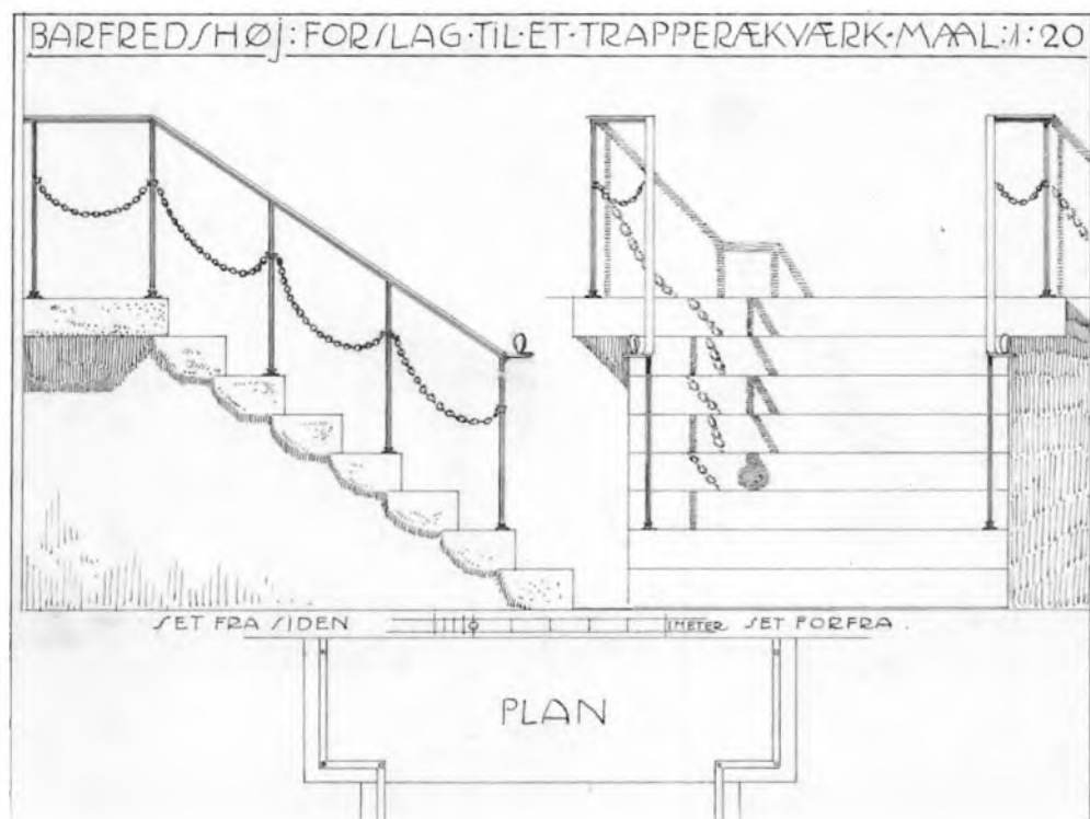
Tegning af nyt gelænder til trappen mod gårdsiden af arkitekt Gerhardt Poulsen 1916
