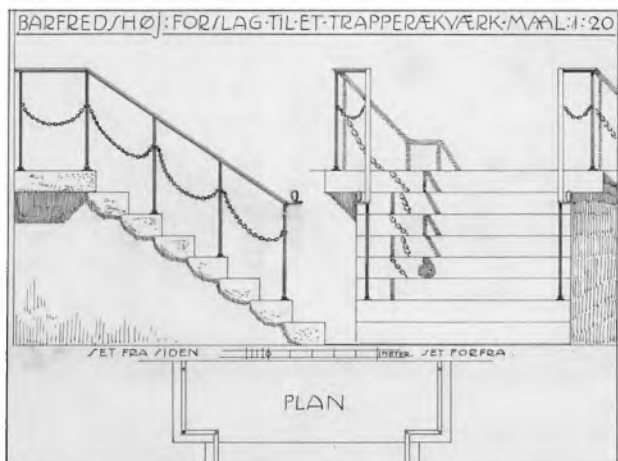
Tegning af nyt gelænder til trappen mod gårdsiden af arkitekt Gerhardt Poulsen
