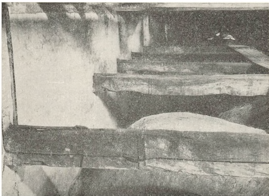
Fig.9 . Loftsbjælkerne i Tamdrup Kirke. Paa Billedet ses 5 af de 7 svære Egebjælker, som stammer fra den oprindelige Søjlebasilika. Under Bjælkerne skimtes Hvælvingerne, som senere er indbygget. (Foto H. Jørgensen).
