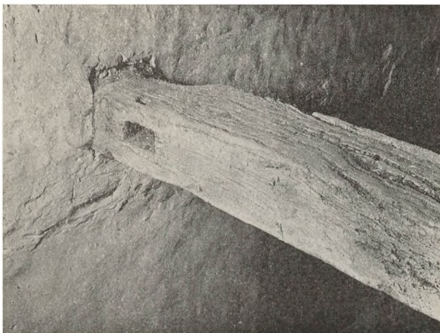
Fig. 11. Bjælke Nr. 7 fra Øst. Stolpehullet i Siden ca. 20 cm fra Væggen vidner om tidligere Brug. (Foto: H. Jørgensen).
