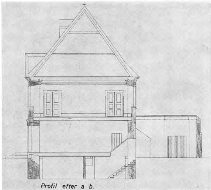
Tværsnit af bygningen.
