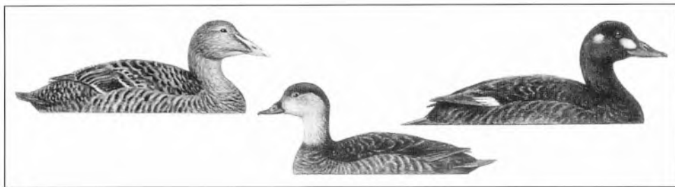
Tre arter af truede danske dykænder, bl.a. i Vadehavet. Det er fra venstre edderfugl, sortand og fløjsand.
