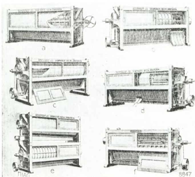
Cylinder- og Centrifugalsigtemaskiner.
