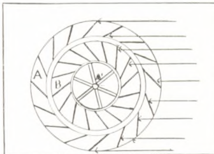
Skematisk Tegning af en horisontal Vindmølle, set fra oven. Man vil se, hvordan de skraat stillede Planer (de mange, tykke Skraastreger) er stillet saadan, at Vinden, hvis Retning vises af Pilene, til den ene Side (Tegningens øverste Halvdel) byder en større Modstand, der fanger Vindkraften, mens den anden Side, der gaar mod Vinden, byder en langt mindre Modstand.
