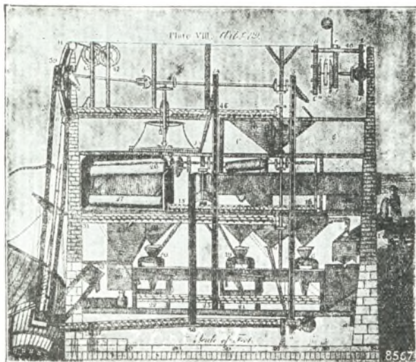
Den automatiske amerikanske Mølle.
