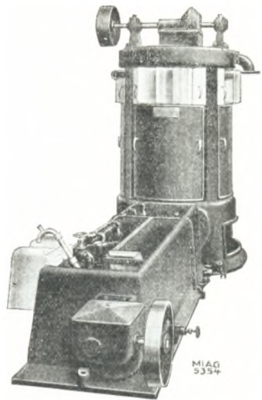
Vaskerianlæg for Korn.
