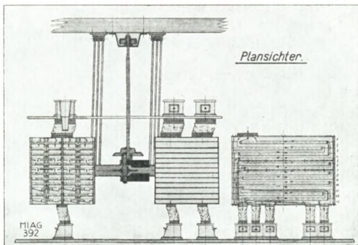
Snit af en fritsvingende Plansigte.
