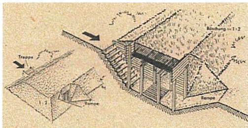
Tegning af den type dækningsgrav der blev bygget på Avnø i sommeren 1941 fra den tyske byggetjenestes (Organisation Todt) vejledning. OT-Lufschutzbauten Heft 1: Ls Gräben.
