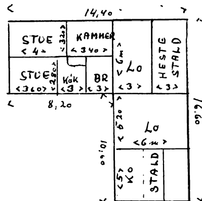
med målangivelse
