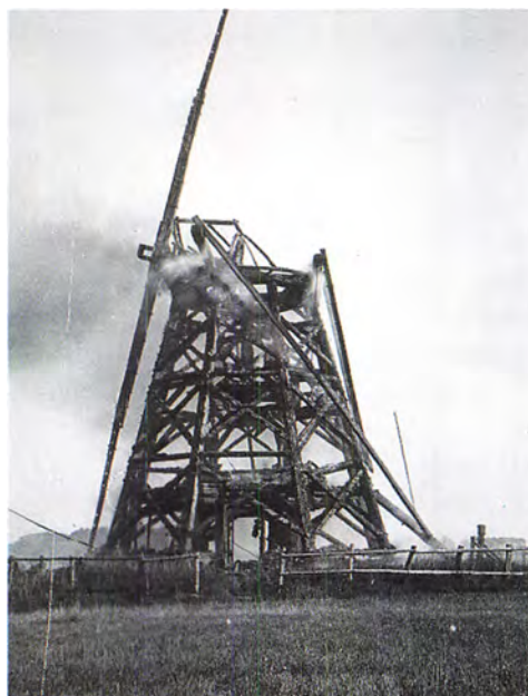
Kysing mølle var en jordhollænder som kunne manøvreres fra jorden. I 1934 brændte den, og stedet mistede samtidig sit sømærke. (Foto: Privatejet).
