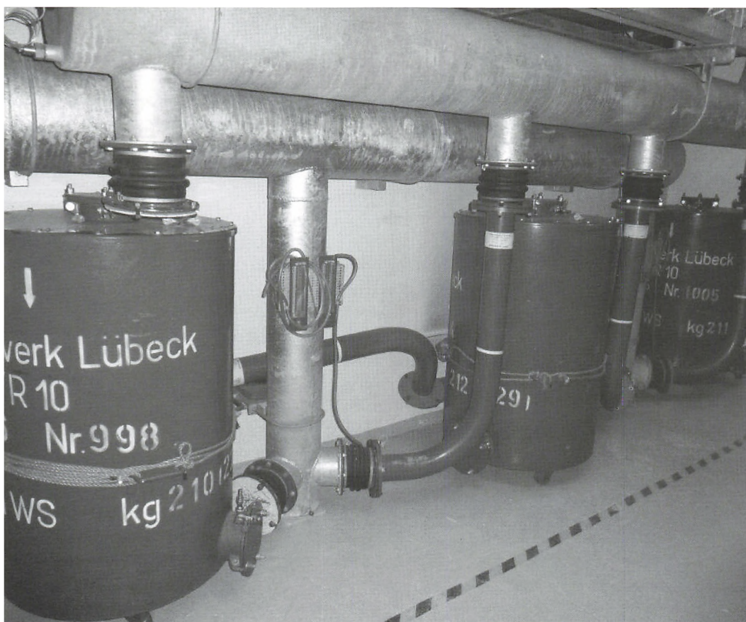
Fig. 9. Gasfilter, der skulle rense luften som blev suget ind udefra. Gasfiltrene er fra det tyske firma Dräger i Lübeck som stadig eksisterer.
