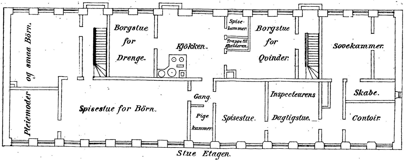
Plantegning af 1. salen og stuen i Røde Bygning efter ændringen 1869/1870 Findes i Johansens beretning fra 1876.
