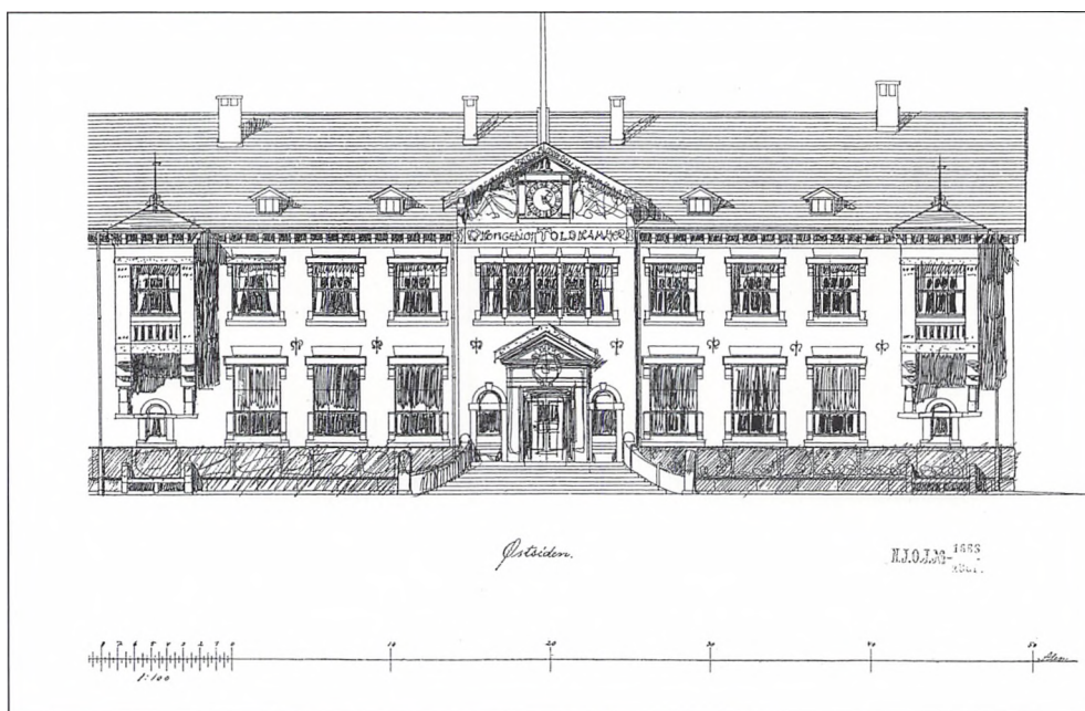
Fig. 94. Ålborg Toldkammer, opført 1900-02 af kgl. bygningsinspektør, arkitekt Hack Kampmann (1856-1920), med det monumentale indgangsparti mod øst. (Tegning af arkitekten i: LAV, Overoldinspektoratet for Nørrejylland, Toldbygninger, 1921-1949 Ålborg (B 297-1.223)).
