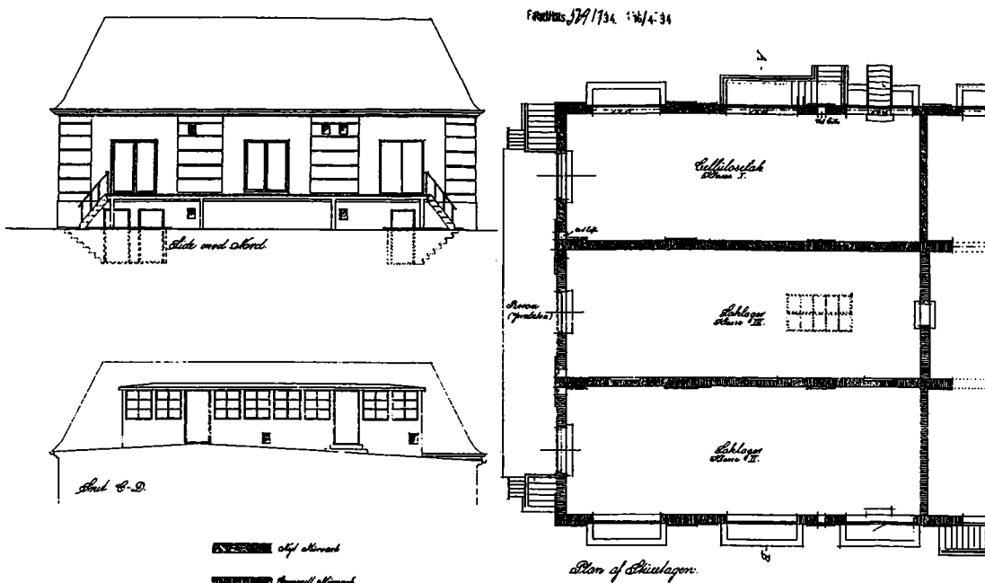
Fig. 75. Udsnit af bygningstegning, der blev indsendt sammen med arkitekt Monbergs ansøgning til Direktoratet for Arbejds- og Fabriktilsynet den 13. april 1934. Tegningsmaterialet omfatter plan- og opstaltstegninger over hele fabrikkomplekset. (RA, Direktoratet for Arbejds- og Fabriktilsynet, Journalsager A 1934 nr. 569).
