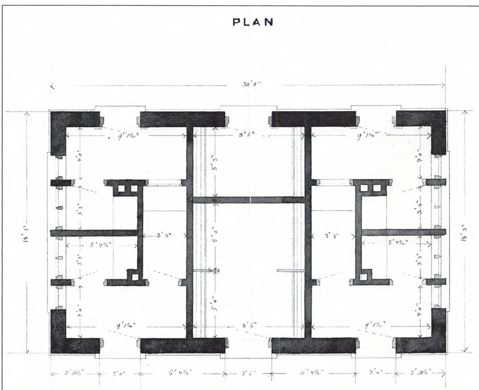
Fig. 53. Tegninger til retirader ved Vendsysselbanen, 1869. Tegningerne omfatter bl.a. et facadebillede og en grundplan. (RA, Danske Statsbaner, Baneafdelingen, Ældre normaltegninger, M VIIb. Tegninger til udhuse, retirader, varehuse og pakrum. Foto: Peter Wodskou).
