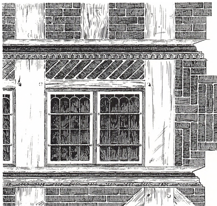
Torammet renaissance-vindue fra et af de nedrevne huse i Bramstræde. Opmåling ca. 1890.
