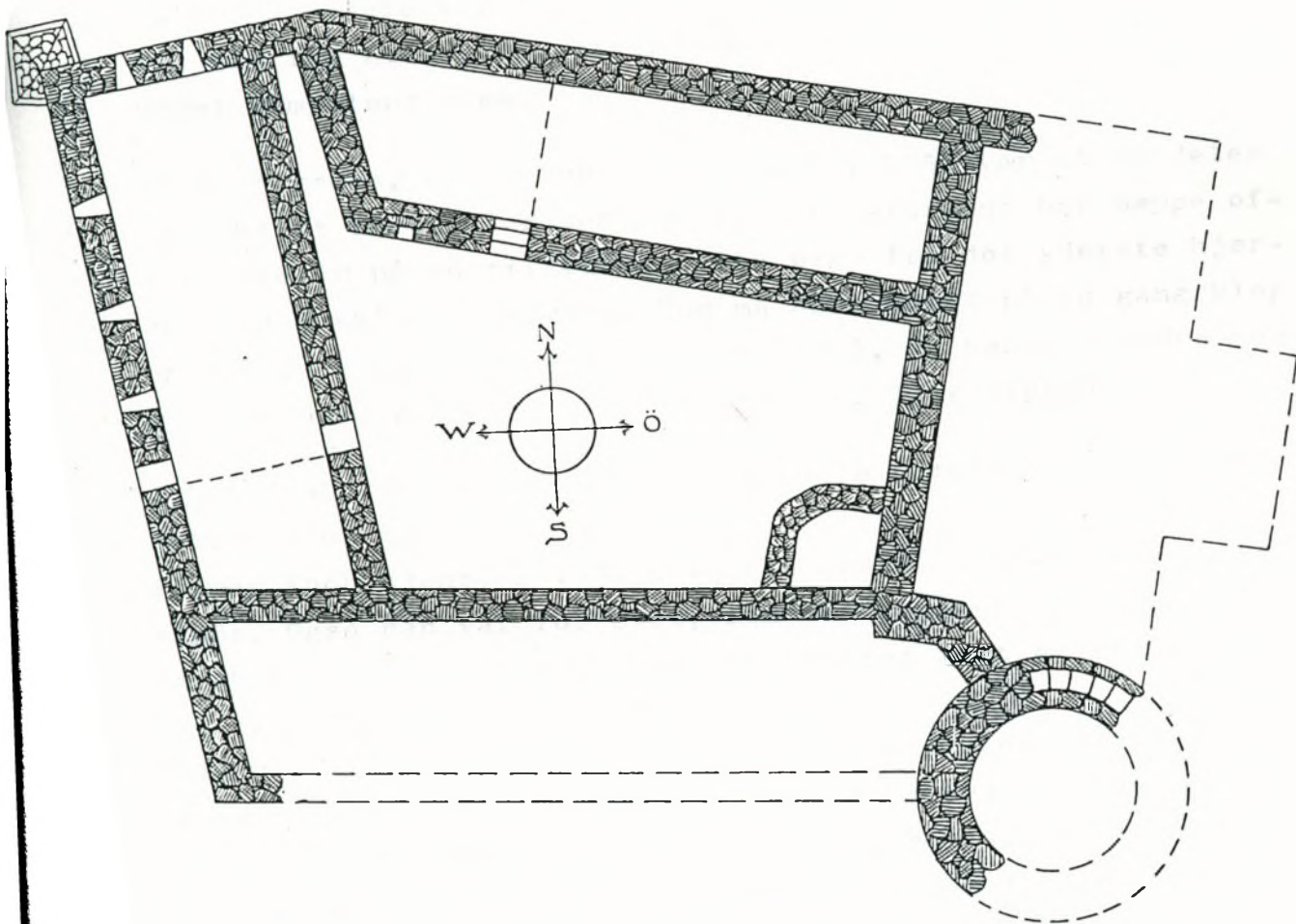
PLAN AV BOTTENVÅNINGEN.
