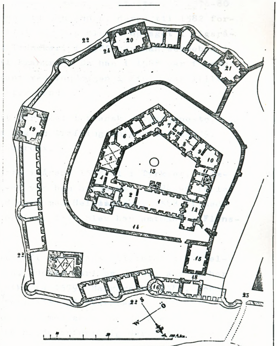
Grundtegning af Hållundborg-Slot.
