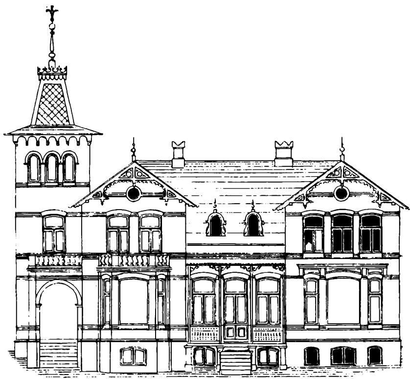
Facadetegning af skibskaptajn Christian Peter Schütts prægtige »Villa Anna Carolina«, der købt af ægteparret Voetmann i 1905 og derefter hed »Haus Ahrensberg« efter bakken, som Aabenraa sygehus står på.
