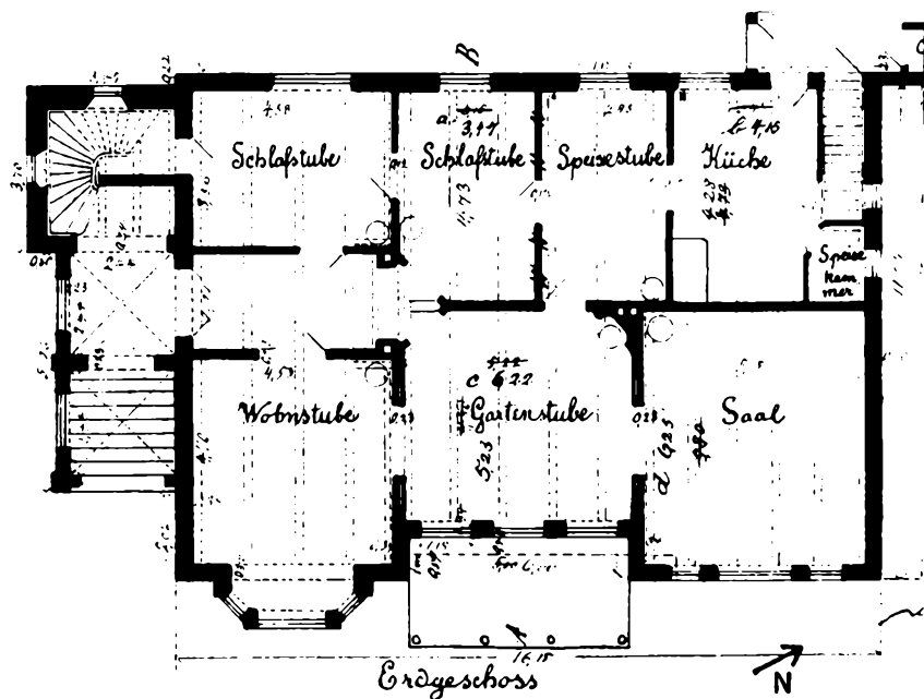
Tegning over »Haus Ahrensbergs« stueetage med tre store stuer på rad.
