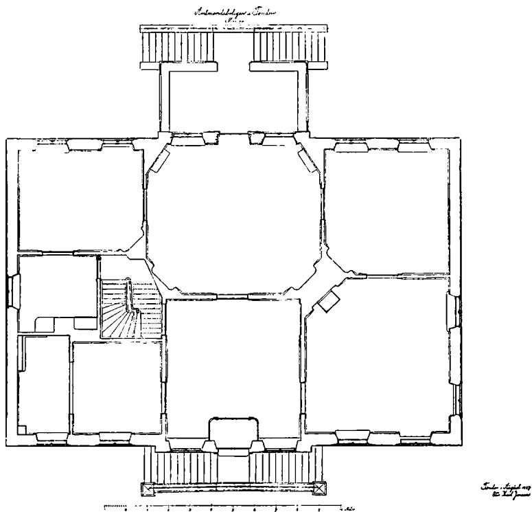
Figur 6: Amtmandsboligens stueetage før 1950 Opmålt af Otto Karl Jensen 1927
