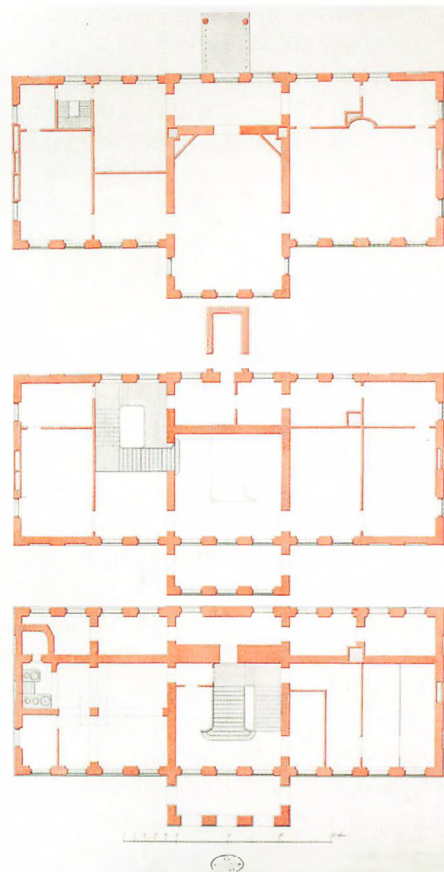
Etageplaner af Marienlyst. Usigneret tegning, vel fra 1700-tallet. Nationalmuseet.
