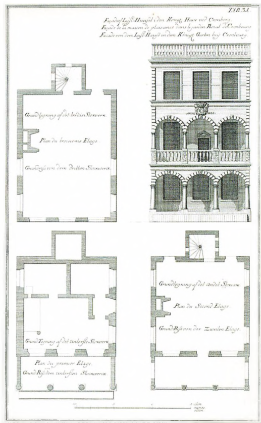
Facade og planer af Lundehave ca. 1750. Efter Lauritz de Thurah: Den danske Vitruvius I-(III) , 1746-(1967).
