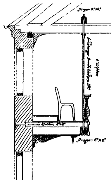
Tegning til balkonen eller galleriet i den store sal. Den hang i jernstænger og var støttet af en gennemgående jerndrager. En trappe førte op til den søndre balkon. Helsingør Kommune. Bygningsinspektoratets arkiv.
