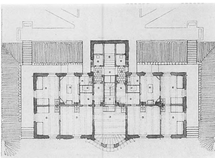
Arkitekt Hans J. Hansens grundplan af husets 2. etage lader ingen tvivl om, hvor sengene skulle stå. Originaltegning i Officershjemmet.
