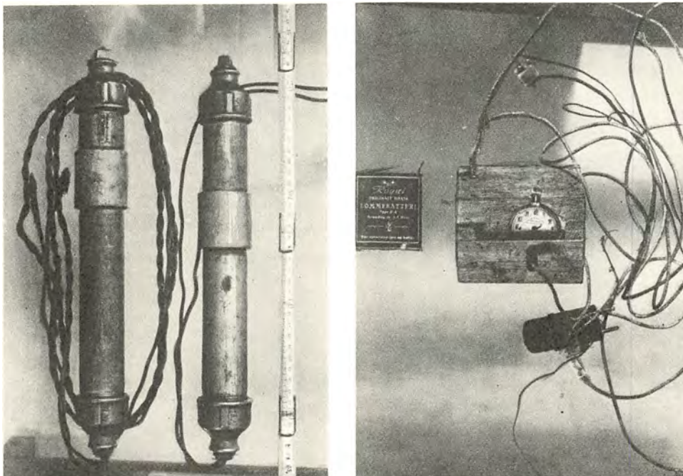
T. v. to hjemmelavede Bomber, hver indeholdende 3 Pakker Aerolit. T. h. Batteri med Lommeur som Tænder. En Ledning gaar til Urets Bagkapsel, en anden til et Bananstik, som berører Urskiven, der er isoleret. Idet den lille Viser naar frem til Bananstikket, sluttet Kontakten. Den store Viser er klippet over, saa der kan opnaas en Tidsindstilling paa ca. 11 \frac{1}{2} Time.
