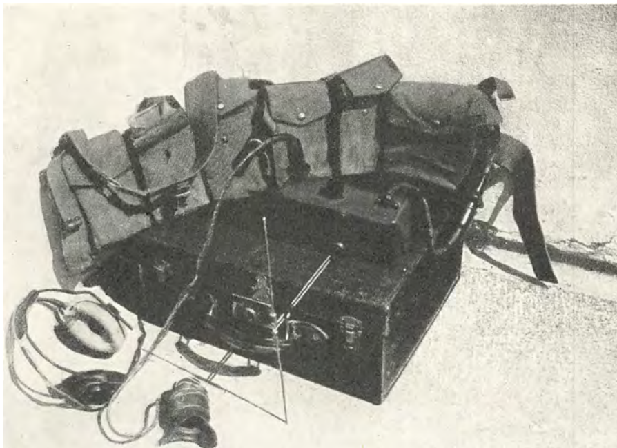
Ved en Radiotelefon som denne var det Mandskabet paa Nedkastningspladsen muligt at samtale med Piloten i Forsyningsmaskinen.
