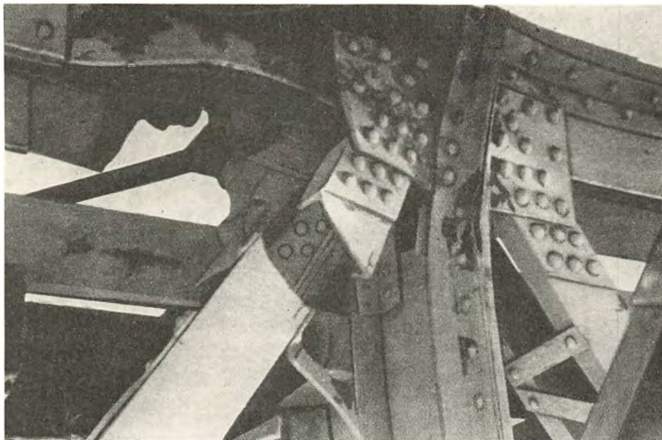
Man gik i November 1943 i Gang med at ødelægge bl. a. de tre Broer over Gudenaen. Her ser man Virkningen paa en af dem. Broen staar ganske vist — men dens Bæreevne er blevet stærkt forringet.
