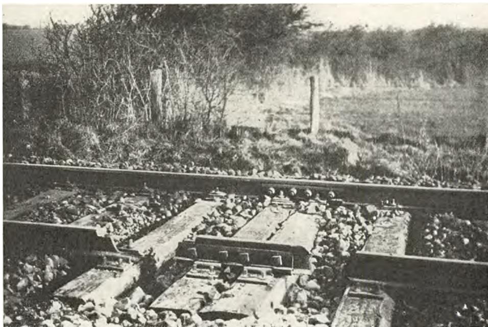
Man har i April 1944 forsøgt at sprænge et af Jernbaneliniens Skinnestød ; men det har vist sig, at der paa Grund af Stødets solide Fastgørelse paa to sammenboltede Sveller har skullet bruges en urimelig stor Sprængladning. Den her voldte Skade har ikke haft praktisk Betydning.
