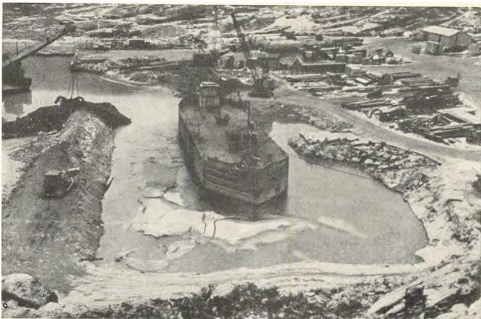
Ved den store amerikanske Hovedbase »Blue West One« indrettede Ingeniørerne ogsaa en Tørdok.
