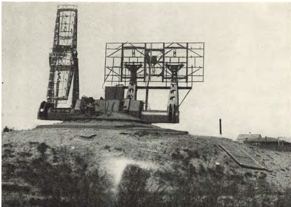
Et af de store, komplicerede tyske Pejleapparater, ved hvis Hjælp man søgte at følge R. A. F.-Maskinerne paa deres Flugt mod Danmark.
