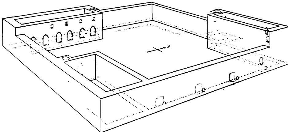
KROGEN SLOT. PERSPEKTIV FRA SYD—ØST
