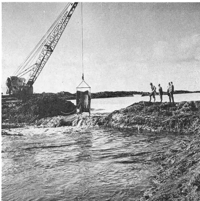
Hver gang en ny strækning af det nye vandløb skal tages i brug, er der spændende øjeblikke. Her æder gravemaskinen sig gennem dæmningen mellem det bagved liggende gamle å-løb — med højere vandspejl — og det nye løb, og millioner af liter vand strømmer ind i det nye løb.
