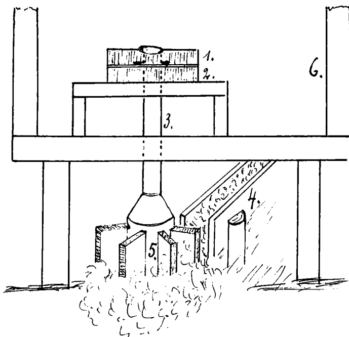
Skitsetegning af en skvætmølle.
