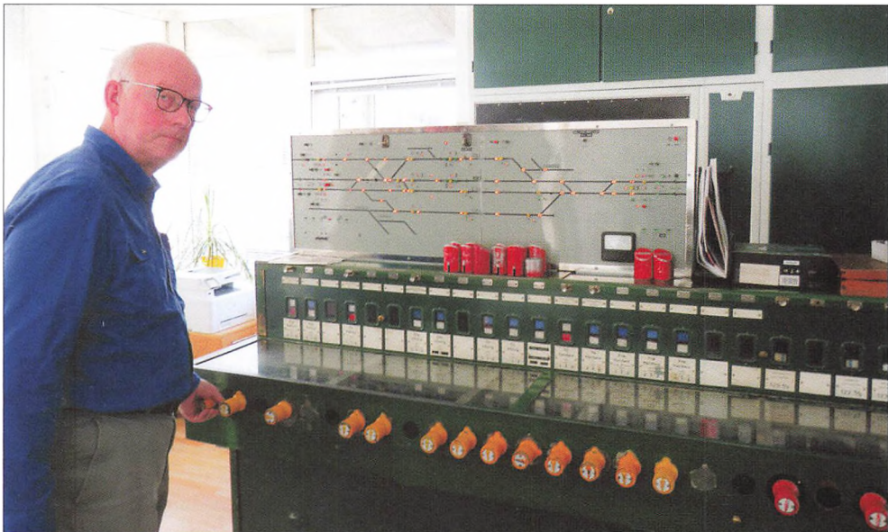
Med bestemte kombinationer af håndtagene stilles sporskifterne i den rette stilling, og når alle betingelser er opfyldt, og alt er gået i hak bag det grønne metal, får togene lov til at køre. Både den grå tavle øverst og de farvede felter over bordet viser tilstandene ude på sporterrænet. Foto: Peter Poulsen
