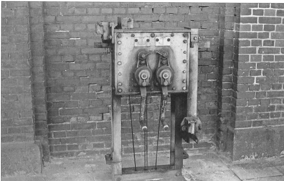
Armsignalerne ved Århus Ø blev betjent fra denne svingbuk, der var placeret på perronen. Svingbukken stod ved hjælp af trådtræk i forbindelse med armsignalerne. Når stationsbestyreren skulle stille signal for et tog, måtte han ud på perronen for at dreje på håndtaget. Når toget var kommet, skulle han huske at dreje håndtaget tilbage igen. Foto: Georg Schmidt.
