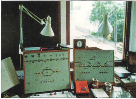
Nye sikringsanlæg blev etableret på stationerne Århus Ø, Torsøvej, Lystrup, Skødstrup og Hornslet. Her ses betjeningsfladen i fjernstyringscentralen i Århus. Foto (arkiv) Georg Schmidt.
