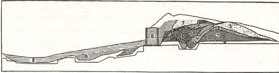
Fig. 26. Skematisk Snit gennem Danevirke. G. Haseloffs Snit ved Rødekro 1936. Tal og Skraveringer angiver sammenhørende Volde og Grave. 1: Ældste Jordvold med Grav mod Syd. 2—4: Senere Udbygning af ældste Vold. 5: Kampestensmuren. 6—7: Udbedringer af denne. 8: Teglstensmuren.
