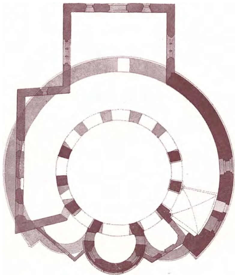
Grundplan af Michaelskirken i Slesvig. Tegning. Nationalmuseet.
