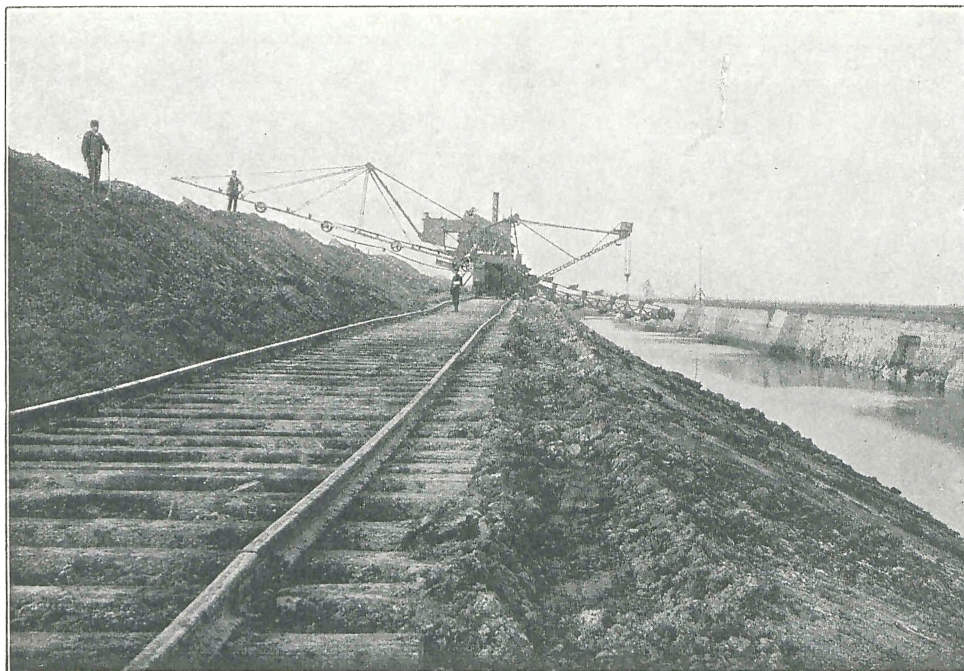
Gravemaskine med indstillelig Transportør. Dige og Fyldgrav. Fra Digeanlægget for Marsken ved Ribe, 1911.
