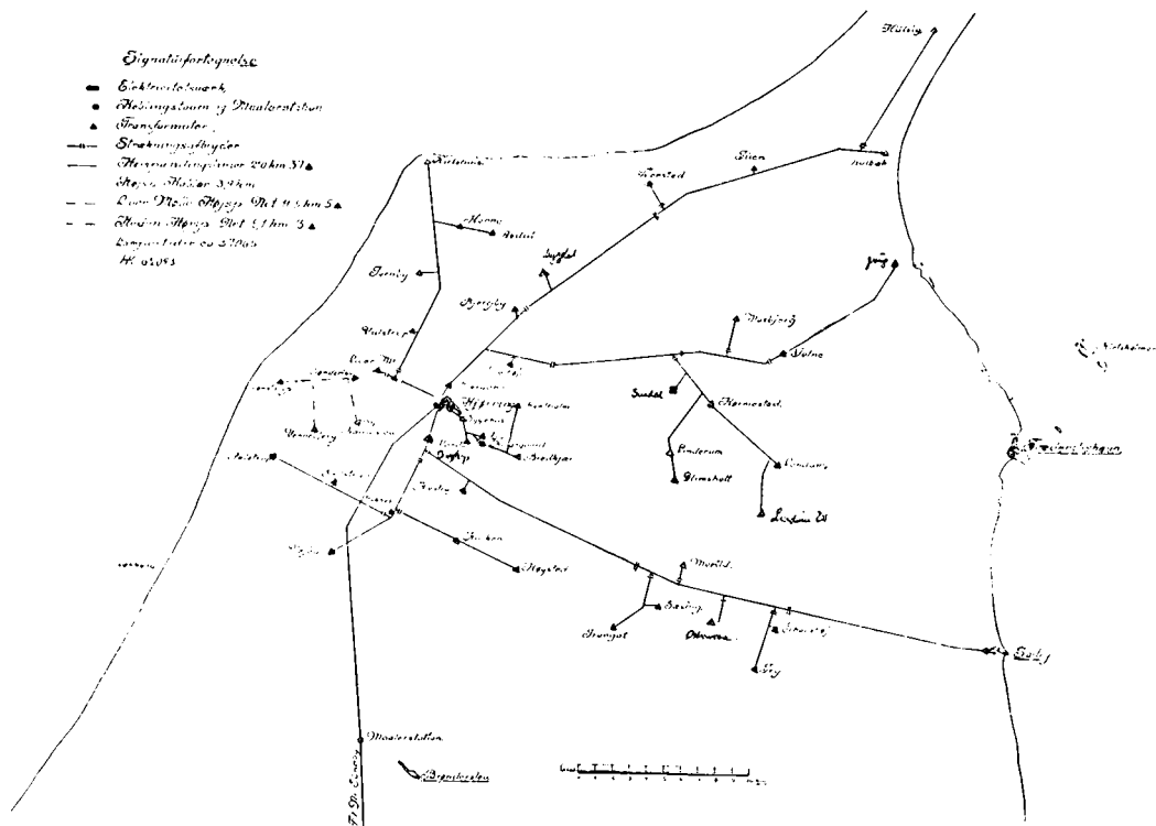
Plan over Hjørring Elektricitetsværks Højspændingsnet.
