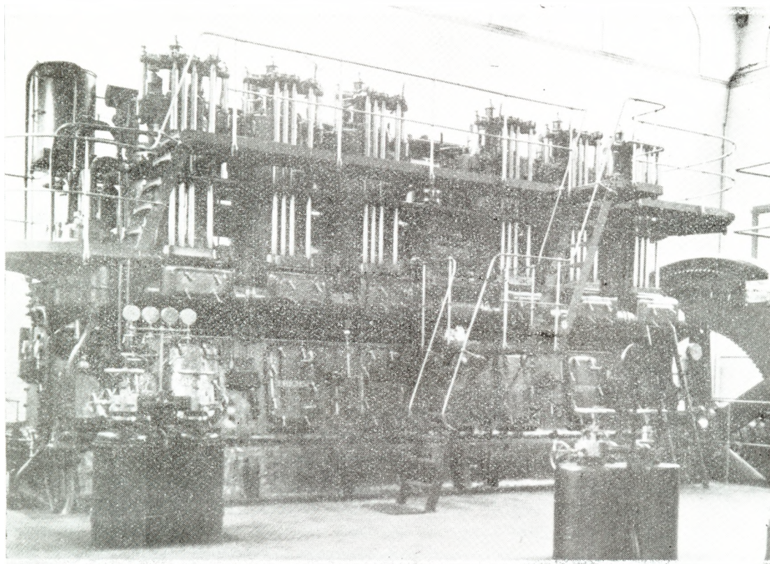
Værkets 6-cyl. 1000 HK. Frichs Dieselmotor.
