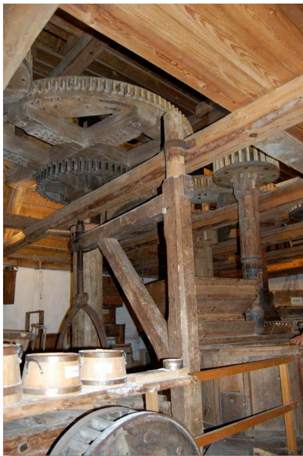
Mølleværket i en vandmølle kører ved hjælp af et sindrigt system af tandhjul – her set på Hjerl Hede.
