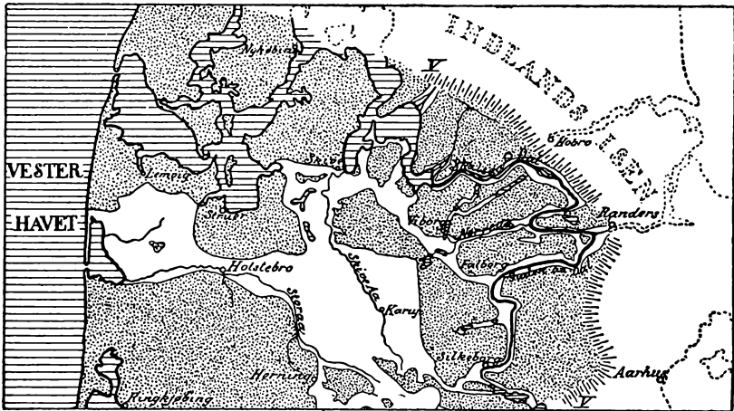
Fig. 3. Iskanten er rykket betydelig længere tilbage mod N. og Ø. og har blottet flere Dale, som saa blev benyttede af Smeltevandsfloder. Smeltevandsfloden fra Silkeborg (Gudenaas Forgænger) søger at trænge ud gennem Randers Fjord, men standses af Isen lidt V. for Randers, saa at den gennem Nørreaa- og Skalsaadalen, maa søge sit Udløb i Hjarbæk Fjord NNV. for Viborg. (Efter Ussing).
