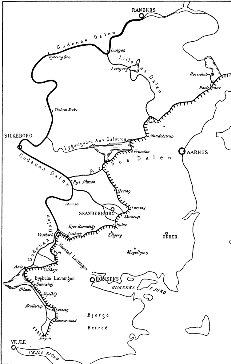
Fig. 4. Kort over Gudenaasens Forgænger, Smeltevandsfloden, som kommer fra Isranden helt nede ved Engom NØ. for Vejle og udmunder i den nu isfri Randers Fjord. Den fuldt optrukne Linie er Gudenaasens Forgænger, Linten med de mange smaa Tværstreger betegner Randen af Indlandsisens under det østjydske Isfremstøds Maximum. Isen dækkede Landet S. og Ø. for Linien. (Efter Poul Harder 1908).
