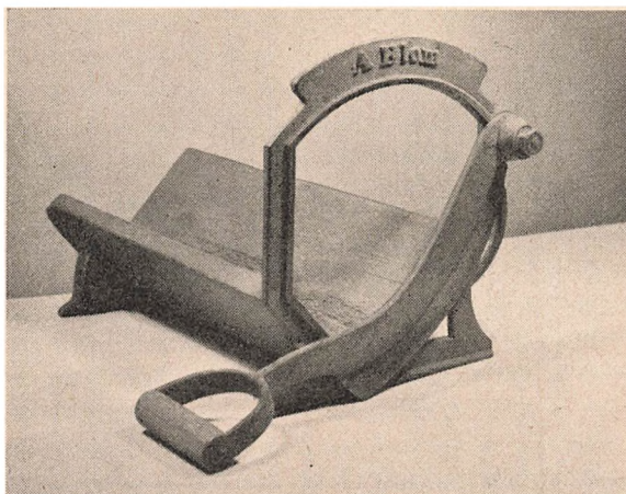
Brødmaskine fra ca. 1868. — Var i Brug paa en Gaard i Illerup 1936 og er brugelig den Dag i Dag.
