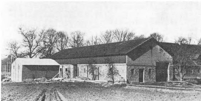
Gammel kampestenslade under ombygning. Hummelballegård. 1965. Laden er opført 1875, kampesten og stråtag. Ændret efter brand 1933: murstensgavl, trimpel og fast tag. 1965 fuldstændig ændring af bygningens indre og ydre.
