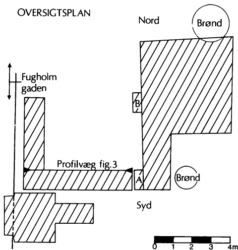
Fig. 2. Oversigtsplan over udgravningen. De undersøgte områder er skraveret. Fugholmgaden ligger til venstre. Profilvæggen fig. 3 samt søjlerne A og B er markeret.
